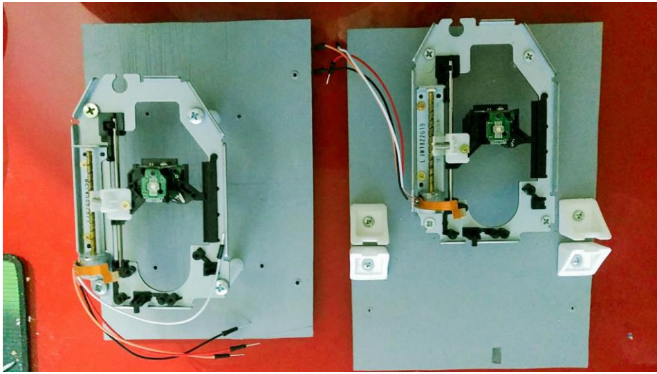
Fig.3 - Os motores de passo aparafusados ao suporte
